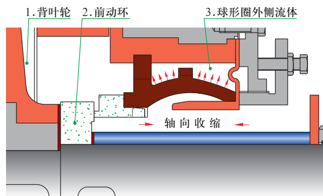
▲ 图二 运行时动静环比压降低原理示意图
