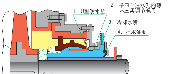
▲ 图十一 冷却系统结构示意图
