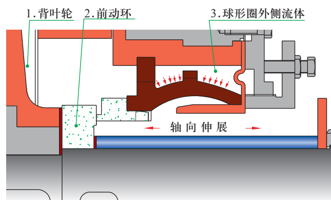
▲ 图三 停车时动静环比压升高不泄漏的原理示意图
