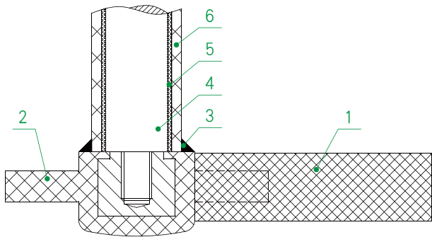
结构简图
