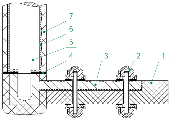
结构简图
